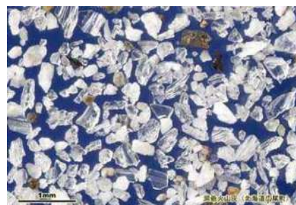
洞爺火山灰の顕微鏡写真
