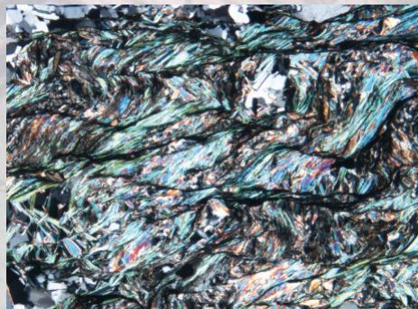
泥質片岩
